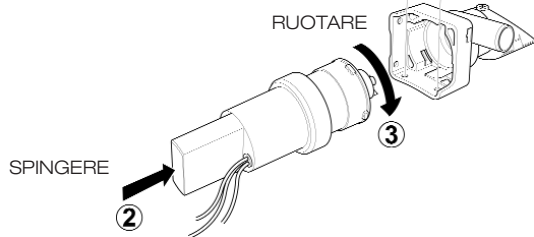
Figura 2 NON avvitare direttamente allo scafo
