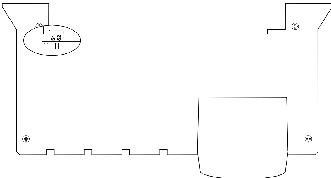
Figure 4: Vue de dessus du convertisseur et position des cavaliers
