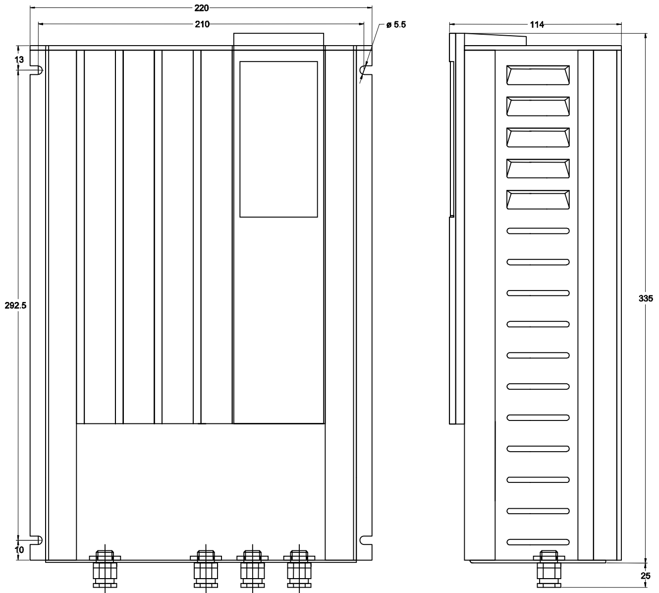
Figure 5: Dimensions du Mass Sine 12/800 - 230V et 24/800 - 230V
