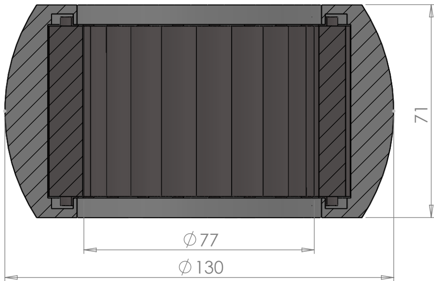
SECTION A-A SCALE 1 : 1.25
