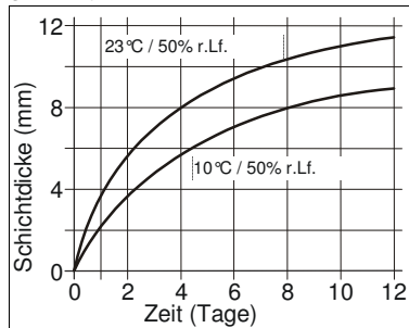
Diagramm 1: Durchhärtengeschwindigkeit für Sikaflex®-221
